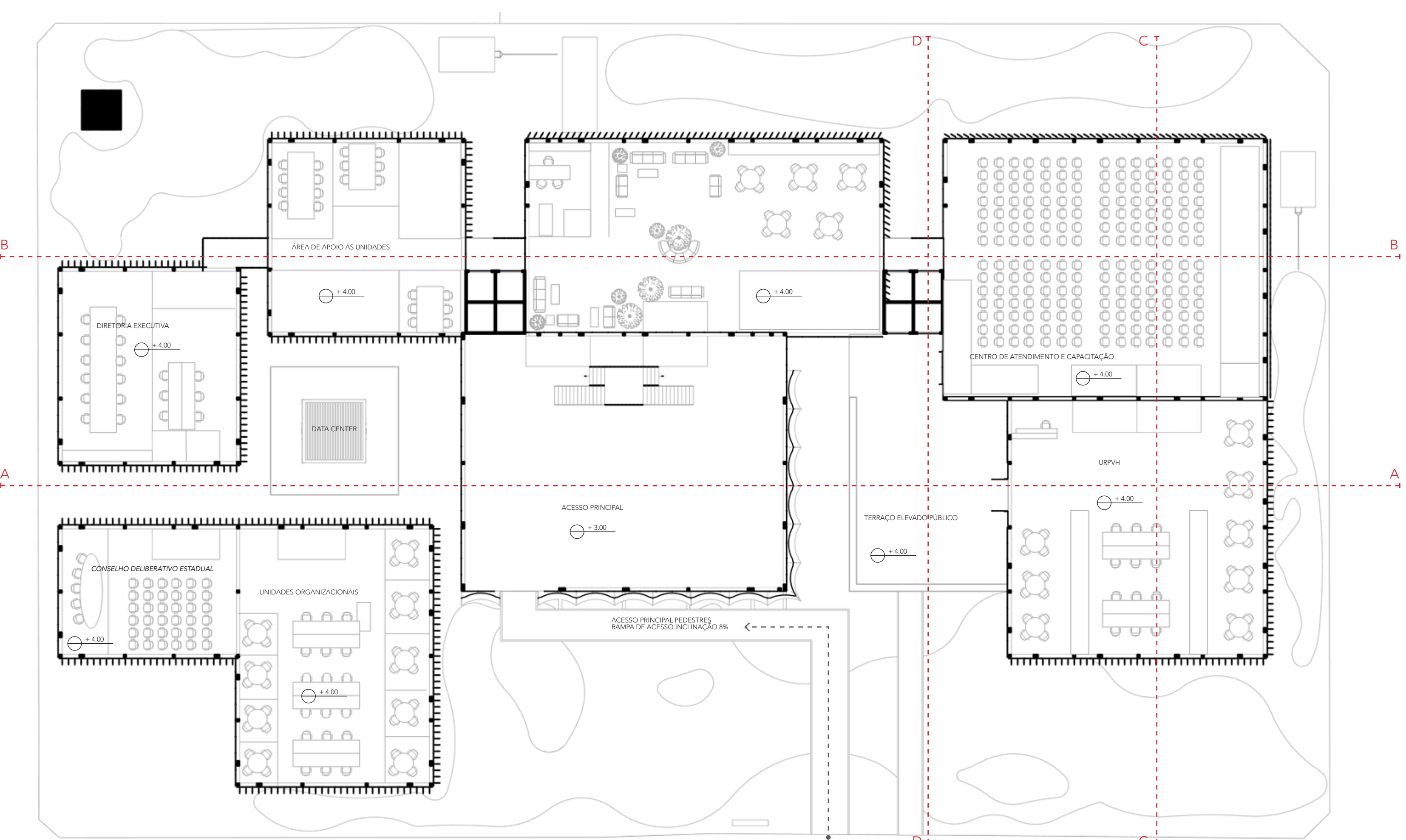
PLANTA PRIMEIRO PAV. - ESC. 1:250
