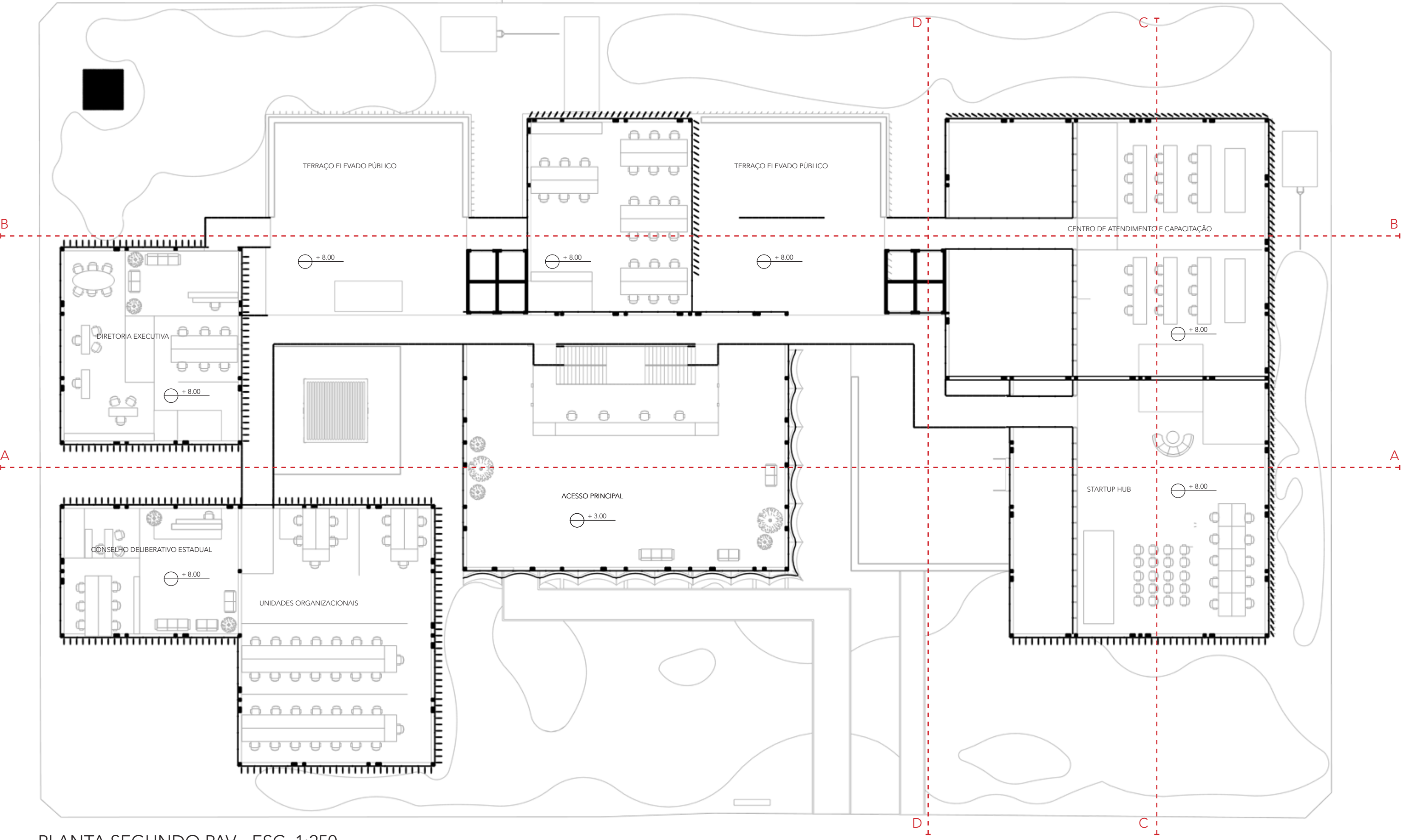
PLANTA SEGUNDO PAV - ESC. 1:250
